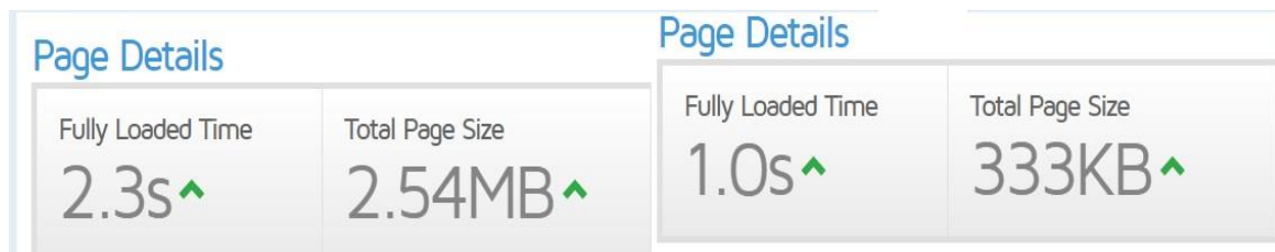
Рис.1.4. Тестування сервісом «GTmetrix» звичайної та AMP-сторінки.
