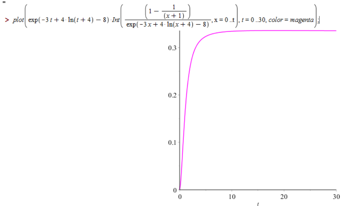
Рис 4. Графік p_0(t) випадок \varepsilon_1(t) = \varepsilon_2(t) = \frac{1}{t+4} .
