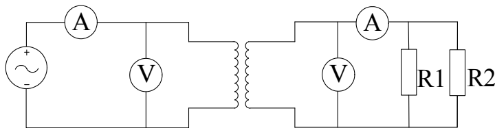
Рис. 7 Додавання споживачів до кола вторинної обмотки трансформатора
