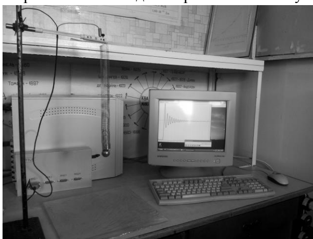
Рис.2. Установа для дослідження зміни напруги на металевій кульці в полі наелектризованої площини з оргстекла
