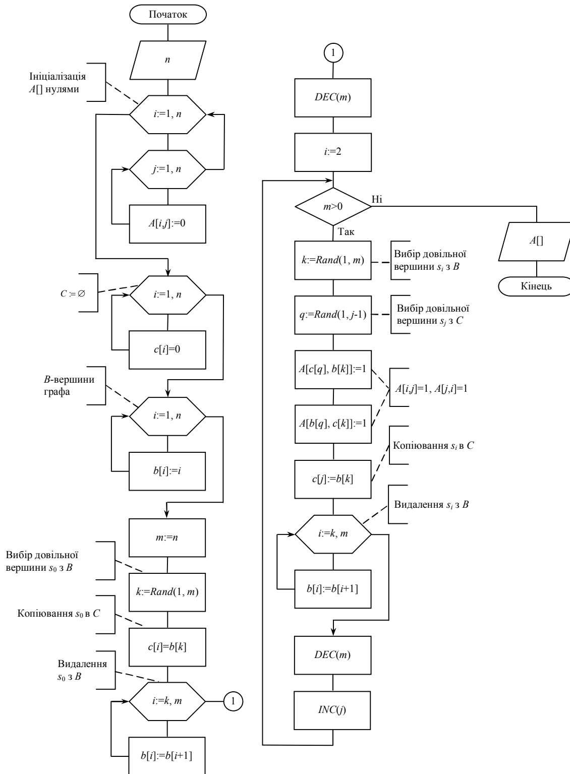
Рис. 1. Блок-схема базового алгоритму генерації дерева
