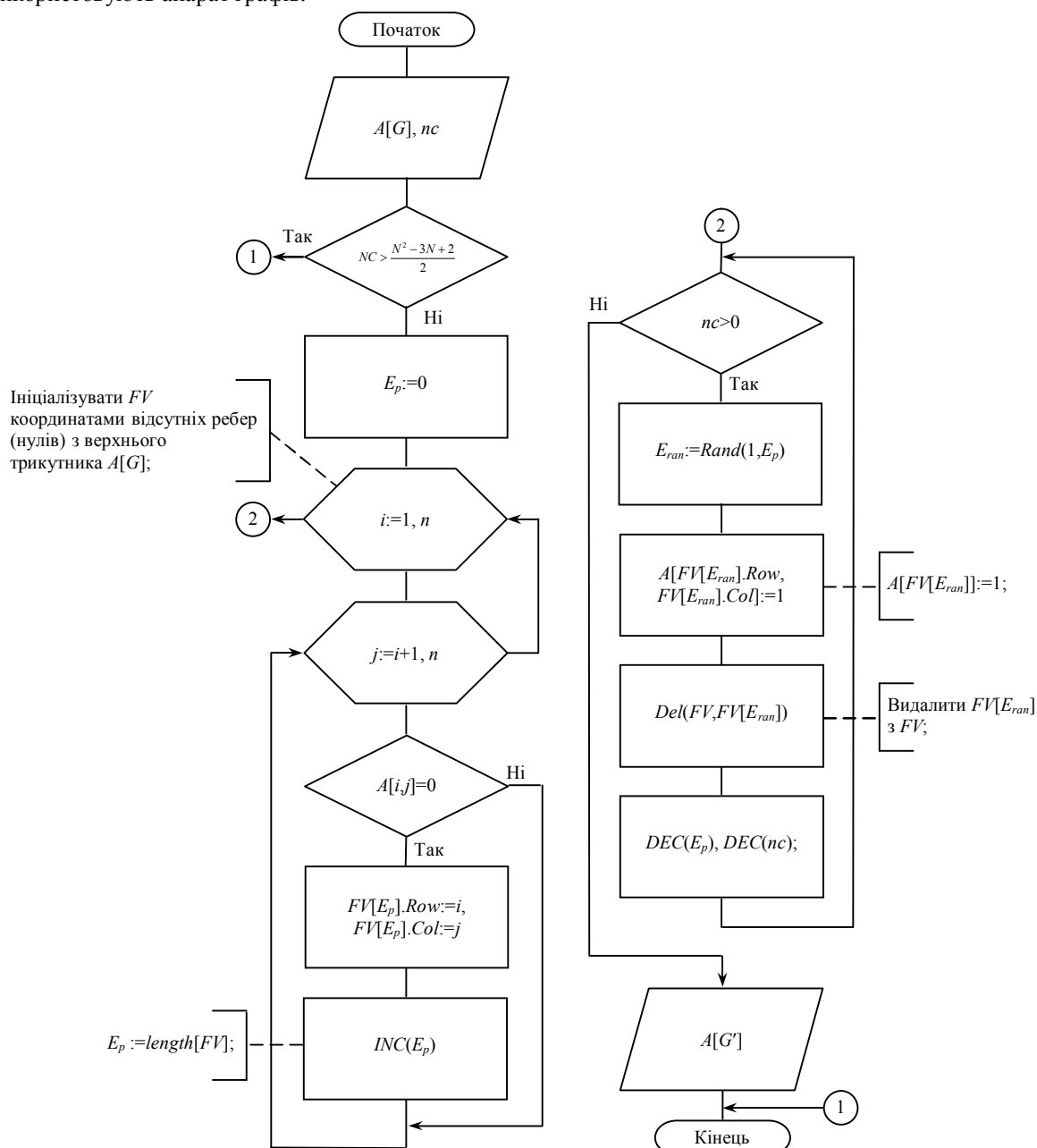
Рис. 2. Блок-схема базового алгоритму генерації графа
